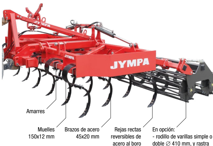
Modelo NEPER-18-3F-PC con rodillo de varillas doble Ø 410 mm
