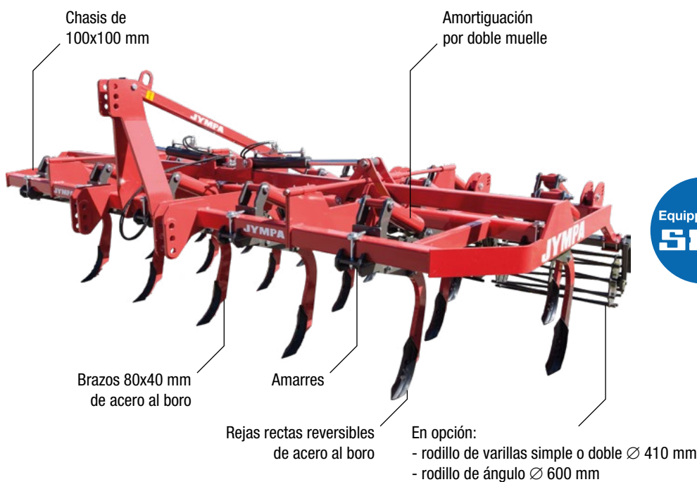
Modelo NIKKAL-17-3F-PL con rodillo de varillas simple Ø 410 mm
