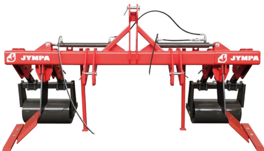
Modelo MINTAKA-2-1800-EH con rodillo liso Ø 325 mm: su chasis extensible hidráulico se adapta mejor a la anchura específica de las calles de los cultivos y aporta más versatilidad.
